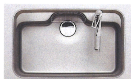
●スキマレスシンク (ステンレスMタイプ) カウンターとの段差が小さく、 継ぎ目の隙間がないので、汚れがたまりにくい。 幅787×奥行最大480/最小403×深さ195mm
